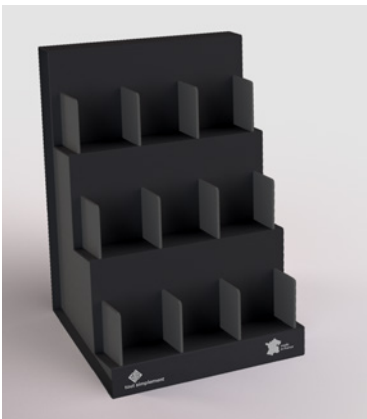
PLV9 / M3.3 présentoir | display avec visuel : H41,5 x L23,5 x P26,5 cm sans visuel : H32 x L23,5 x P23,5 cm 9 emplacements | 9 slots capacité | capacity 108 pcs (9x12pcs)
